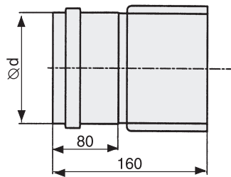
Патрубок для прохода через стену Код: 2400-Ø-WF
