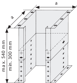
Цокольный элемент, гибкий Код: 2250-Ø-SV
