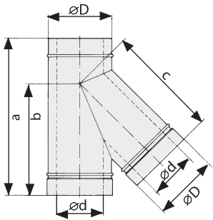
Патрубок к газоотходу 45° Код: 2250-Ø-F45
