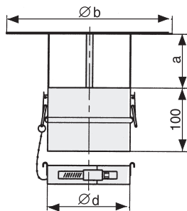
Зонт Код: 2400- \varnothing -RH
