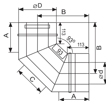
Отвод 93° Код: 2250-Ø-B93
