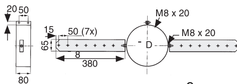
Стропильное крепление Код: 2250-Ø-S
