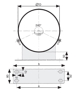
Настенный кронштейн Код: 2250-Ø-W
