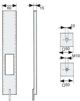
Опорная шина Код: 2400-Ø-AS
