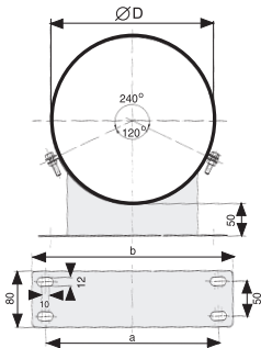
Настенный кронштейн Код: 2400-Ø-W
