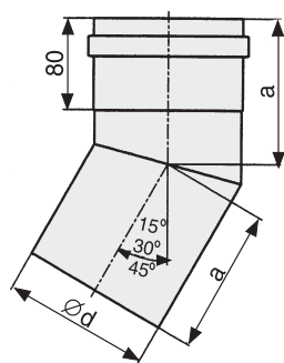
Отвод 15°, 30°, 45° Код: 2400-Ø-B15, 2400-Ø-B30, 2400-Ø-B45
