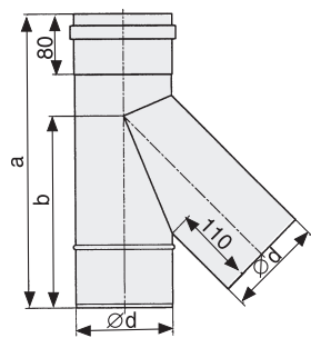
Патрубок к газоходу 45° Код: 2400-Ø-F45
