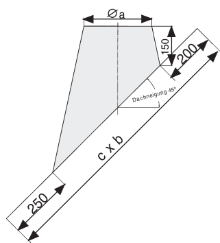
Разделка крышная, наклонная 45° со свинцом Код: 2250-Ø-DGB45
