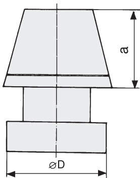
Оголо́вок с кони́ческим заверша́ющим элементом Код: 2250-Ø-AK
