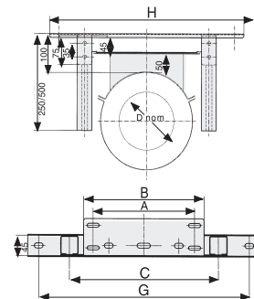
Настенный кронштейн, регулируемый 100-500 мм Код: 2250-Ø-WVLL
