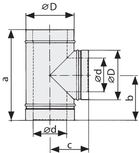
Патрубок к газоотходу 90° высокие температуры Код: 2250-Ø-F90H
