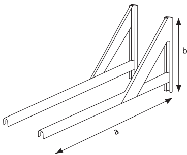
Удлиняющий элемент настенной консоли, гибкий 50-500 мм, 50-250 мм Код: 2250-Ø-WKVL, 2250-Ø-WKVK
