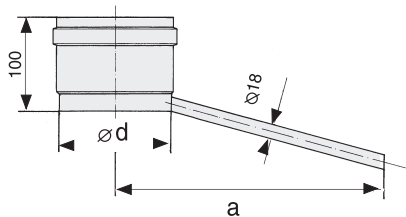
Конденсатосборник с конденсатоотводчиком Код: 2400-Ø-K
