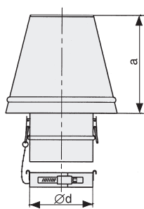
Оголовок Код: 2400- \varnothing -AK
