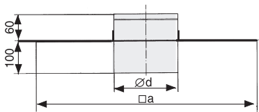
Завершающий элемент Код: 2400-Ø-АЕ
