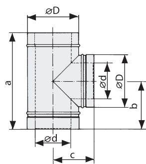
Патрубок к газоотходу 90° низкие температуры Код: 2250-Ø-F90N
