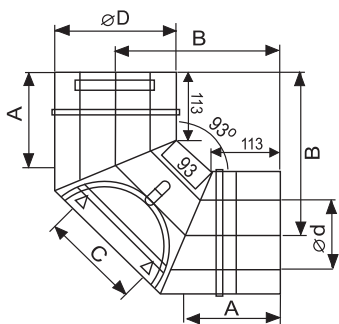
Отвод 93° с окошком для осмотра и прочистки Код: 2250-Ø-BP93
