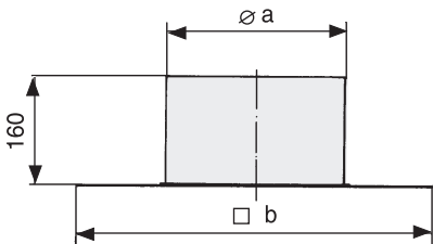
Огнеупорная разделка Код: 2250-Ø-BS
