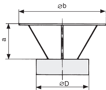
Козы́рек с заверша́ющим элементом Код: 2250-Ø-RH
