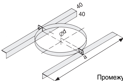
Промежуточная опора Код: 2400-Ø-ZS
