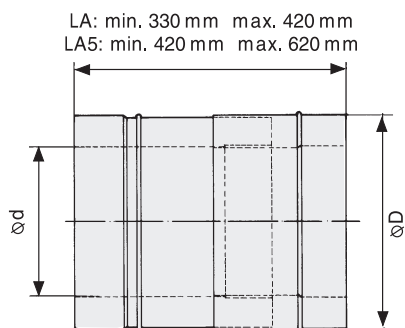
Компенсационный отрезок трубы Код: 2250-Ø-LA, 2250-Ø-LA5
