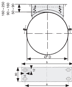
Настенный кронштейн, регулируемый Код: 2250-Ø-WHV, 2250-Ø-WHV9, 2250-Ø-WHV16, 2250-Ø-WHV25
