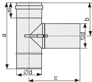
Патрубок к газоходу (тройник) 90° для низких температур Код: 2400-Ø-F90
